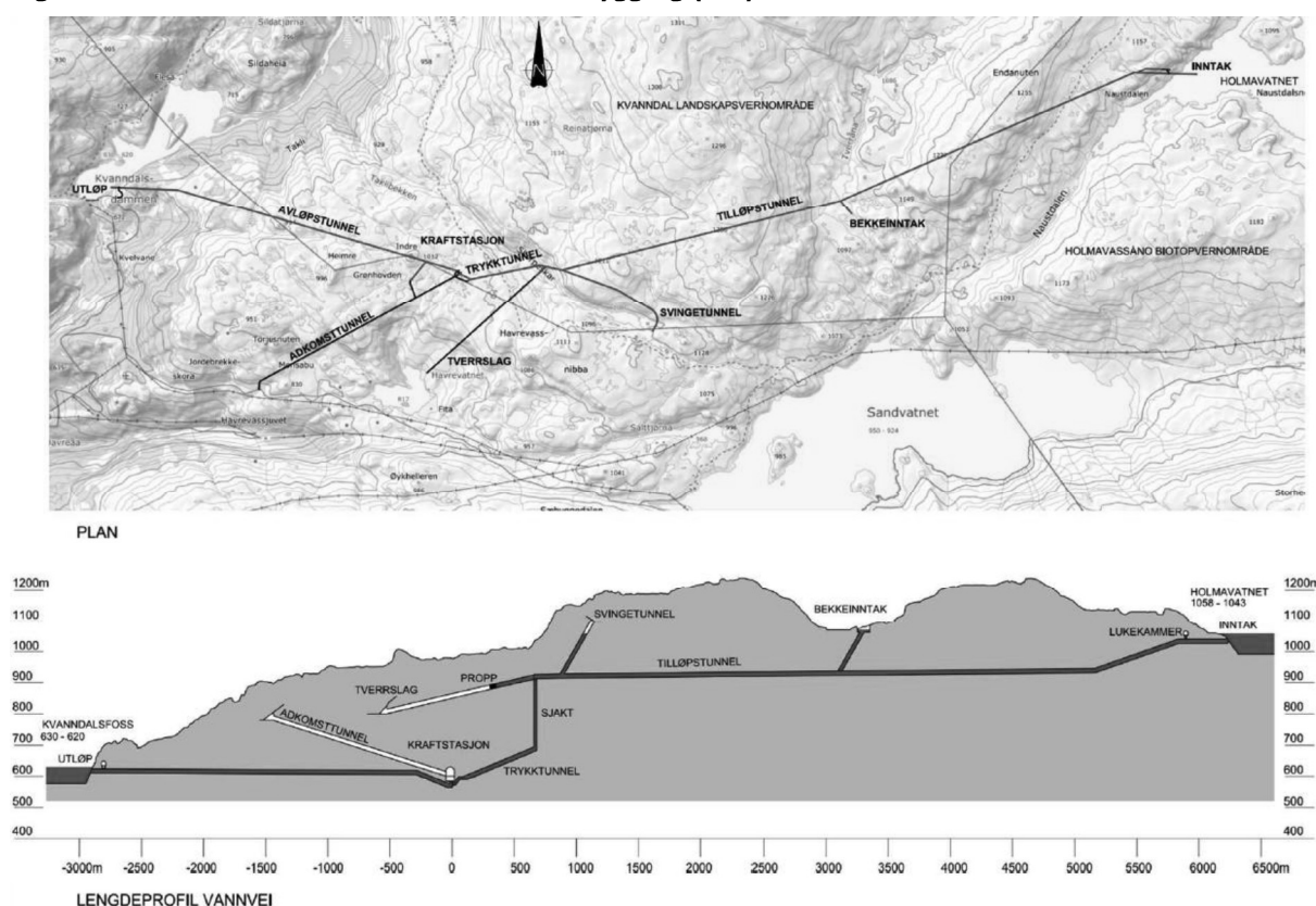
Figur 4. Kraftverkene i Øvre Suldal etter utbygging (OU).
