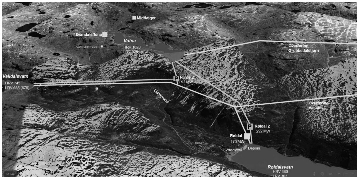
Figur 7 Kraftverkene i Røldal etter utbygging (OU).
