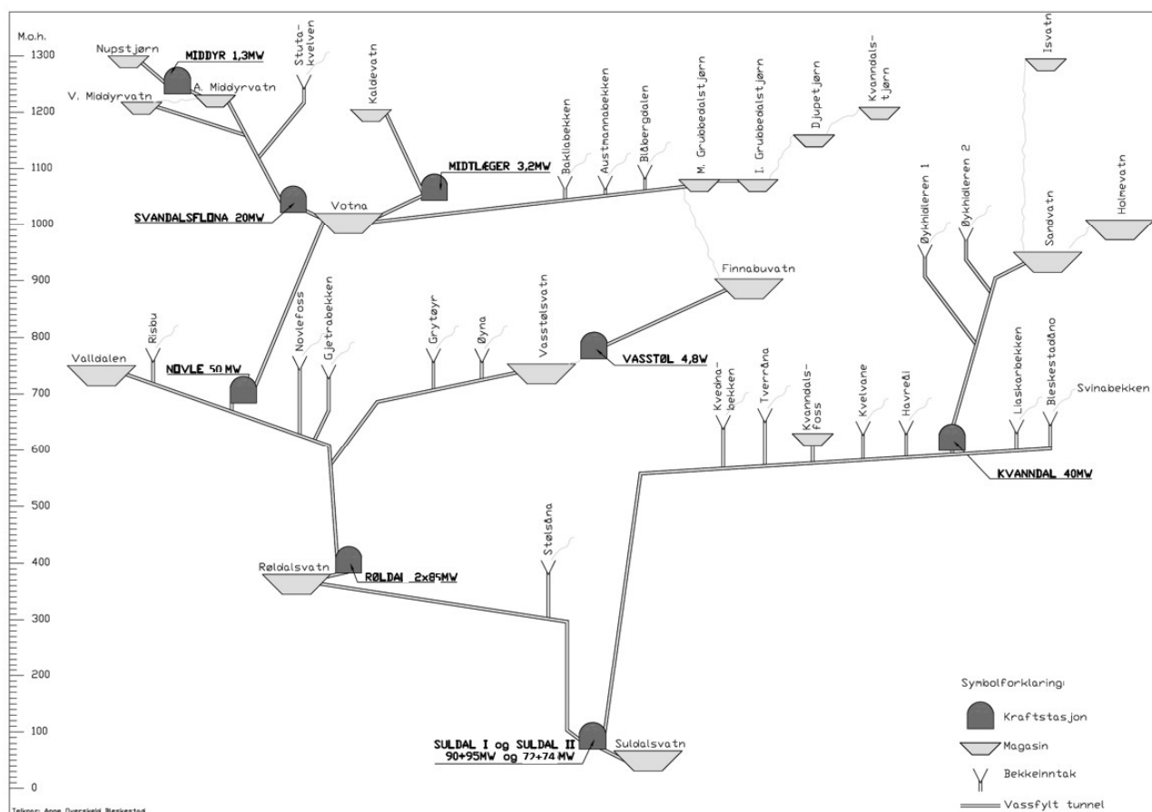
Figur 4-2 Prinsippskisse av Røldal – Suldal anlegga. Sjå større versjon i Vedlegg 2.
