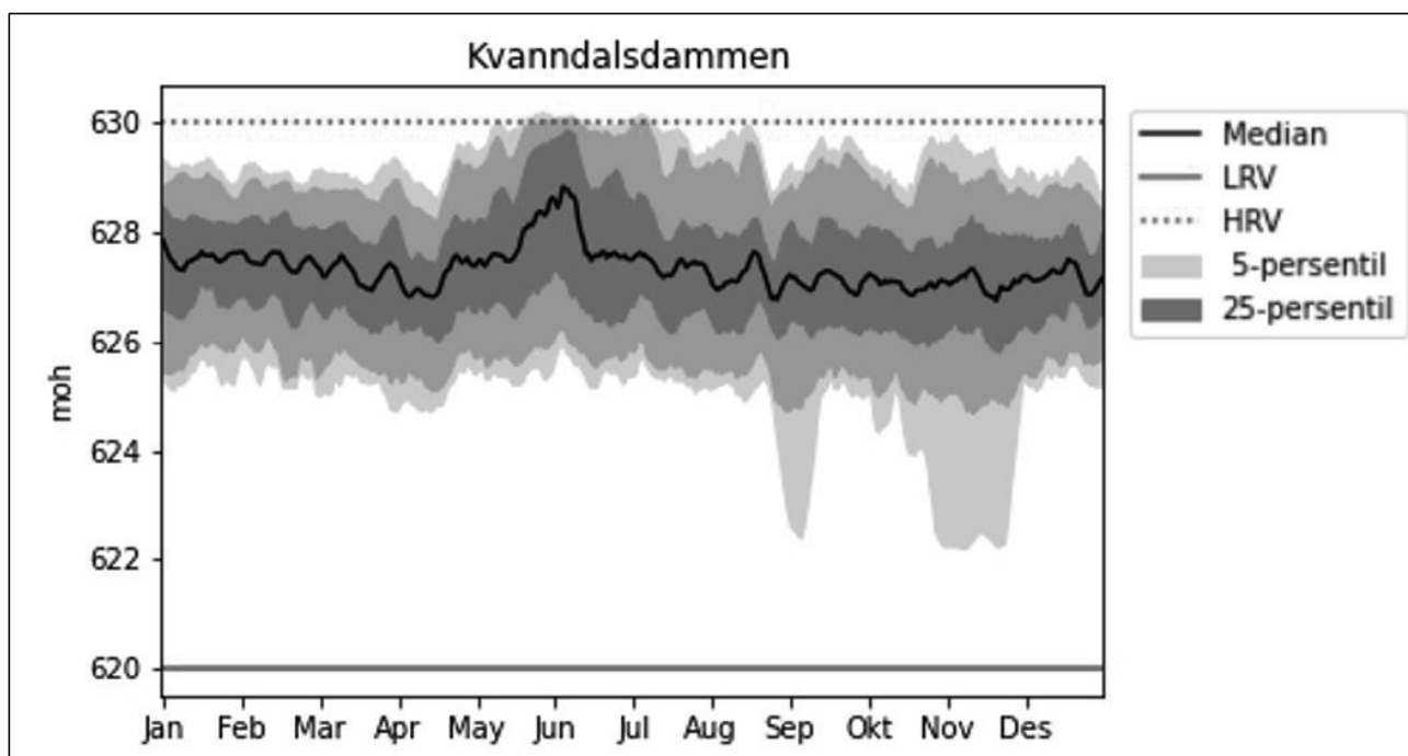
Figur 7-3 Magasinfyllingskurve for Kvanndalsfossmagasinet.
