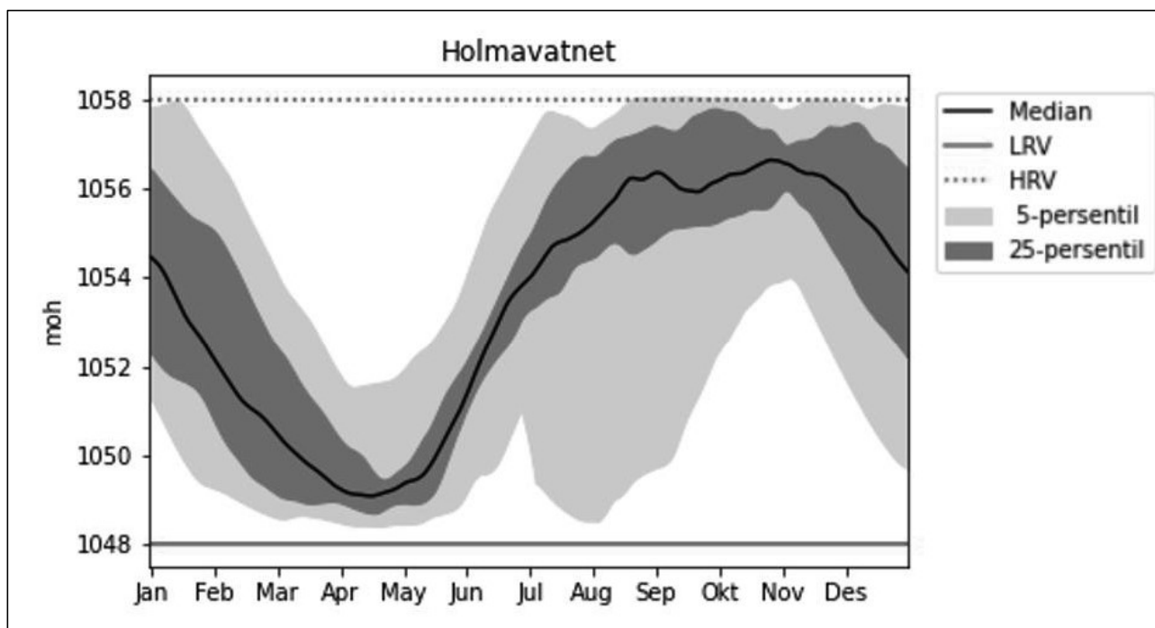
Figur 4-6 Døme på kurve for magasininfylling - Holmavatnet. Tilsvarande kurver for alle magasin ligg i Vedlegg 4.
