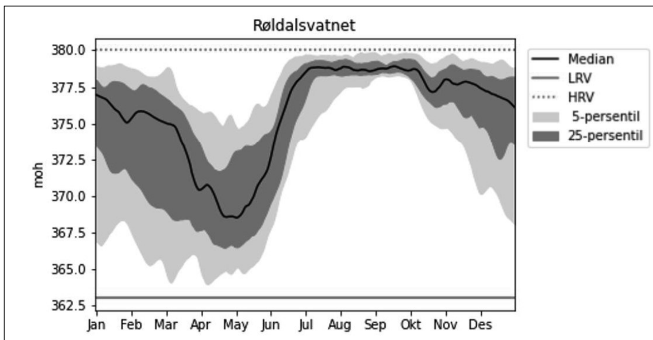
Figur 7-2 Magasinfyllingskurve for Røldalsvatn.
