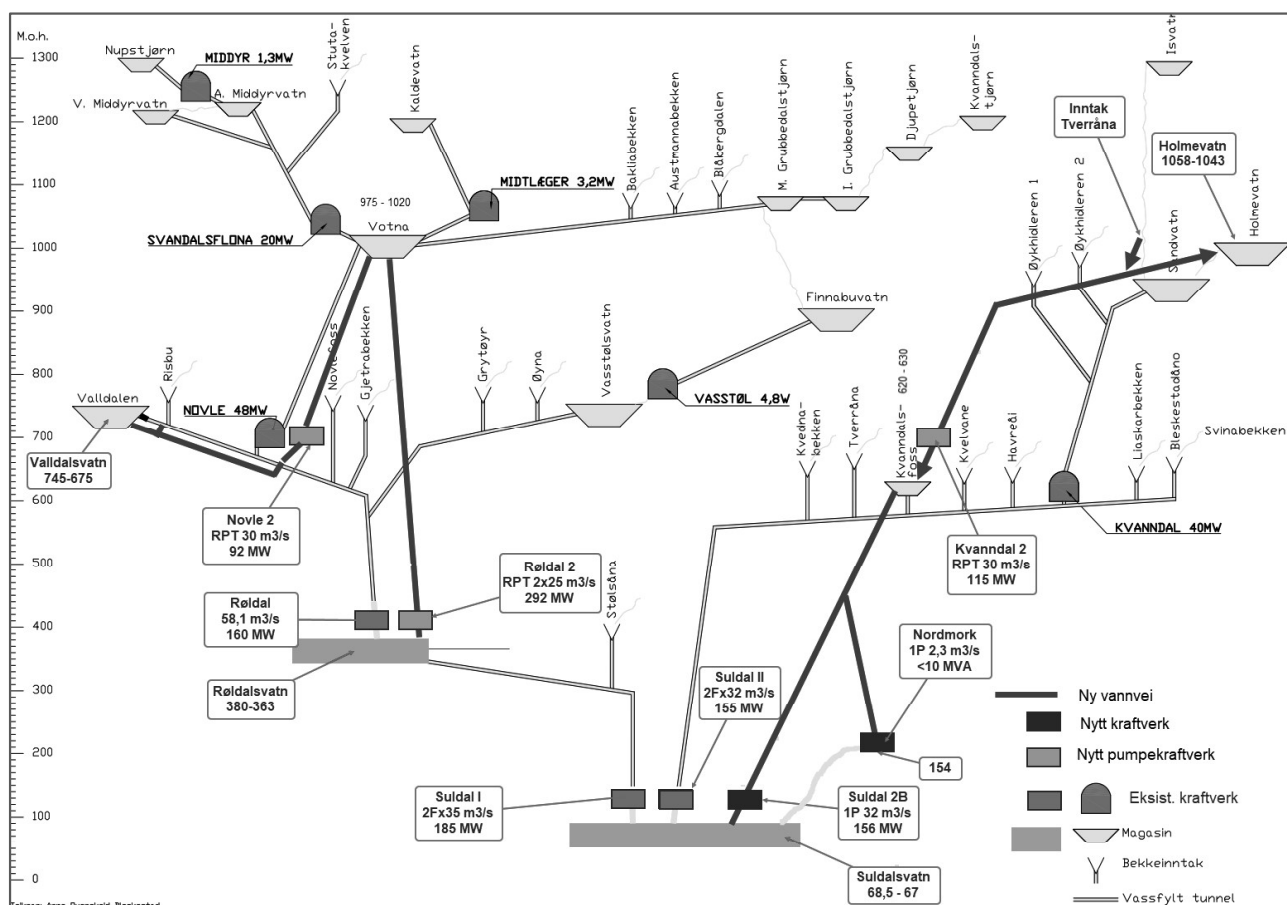
Figur 10-2: RSK OU. Utbyggingsplan skjematisk vist i vertikalplanet.
