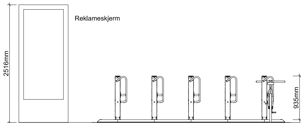
SNITT, SETT MOT NORDØST
