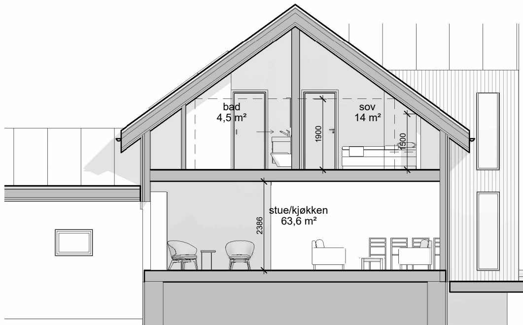
Snitt F 1 : 100
