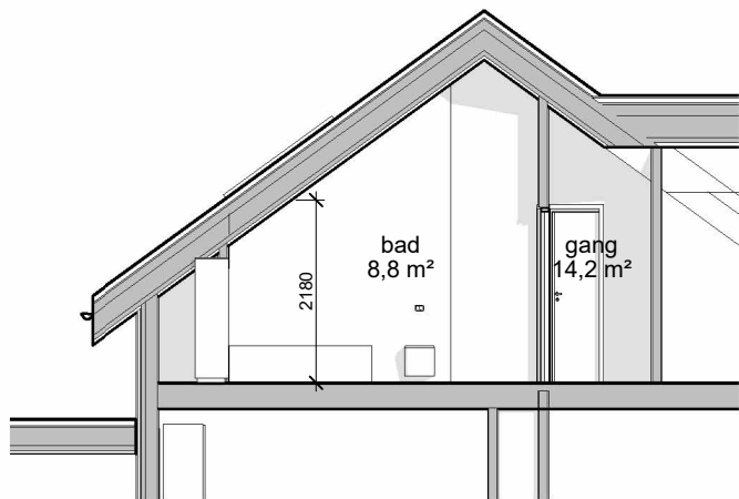
Snitt D 1 : 100
