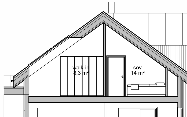
Snitt E 1 : 100
