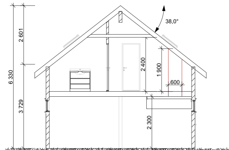
Snitt A-A
