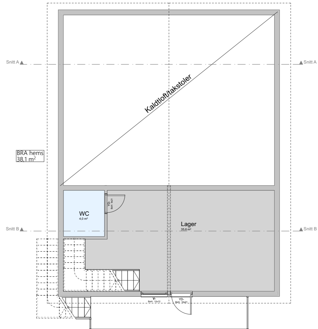
Hems 1:100
