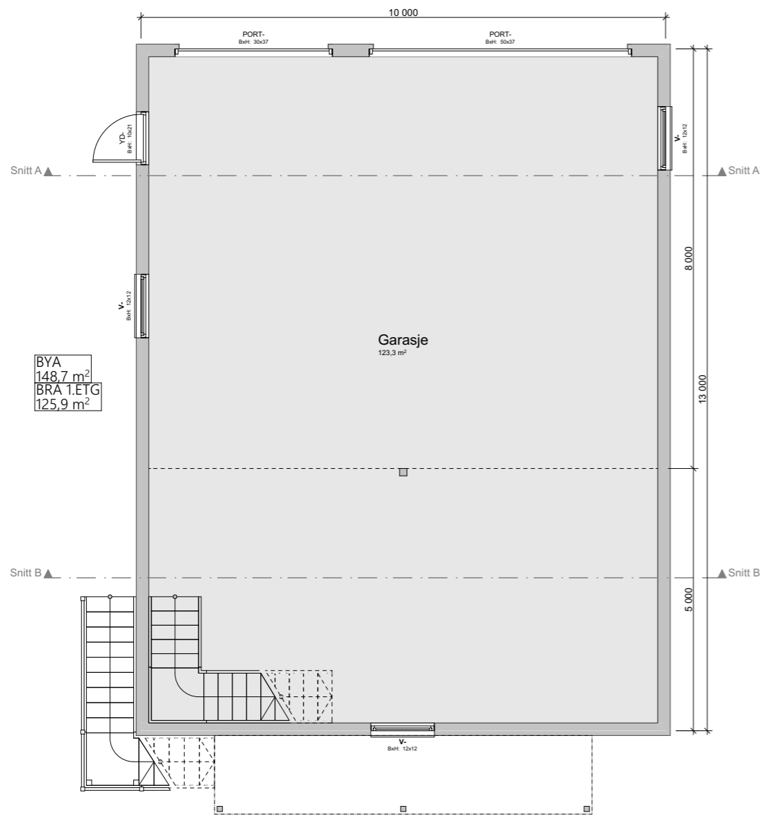
1. etasje 1:100
