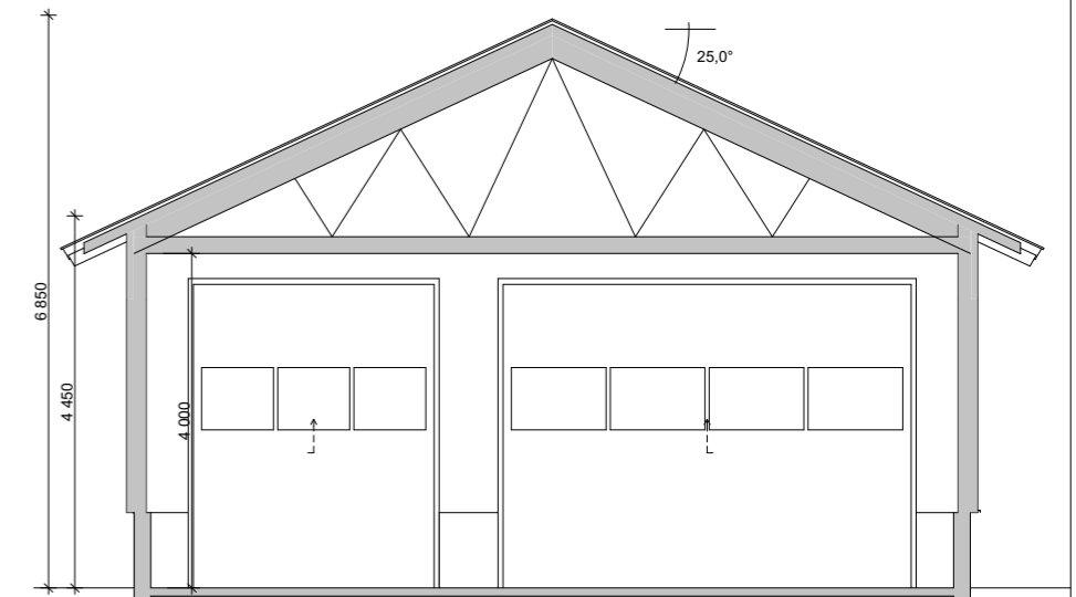
Snitt A 1:100
