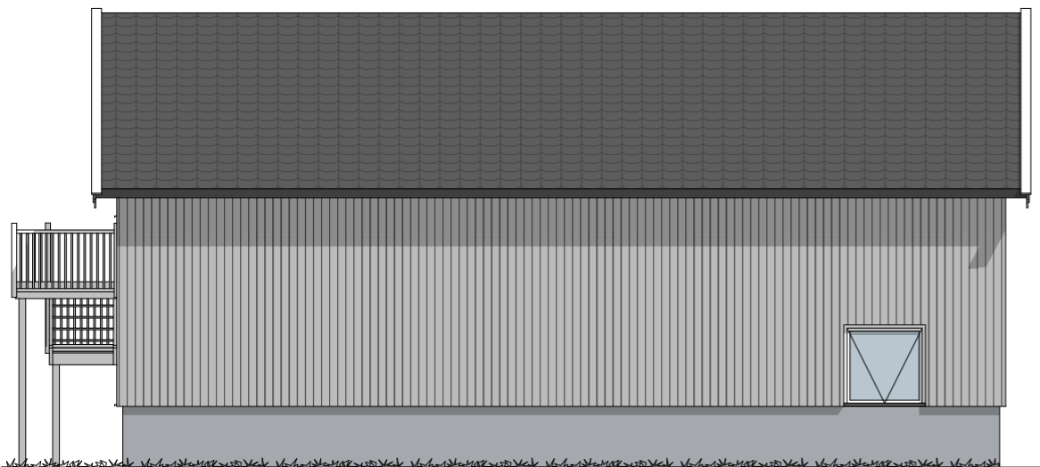
Fasade Øst 1:100
