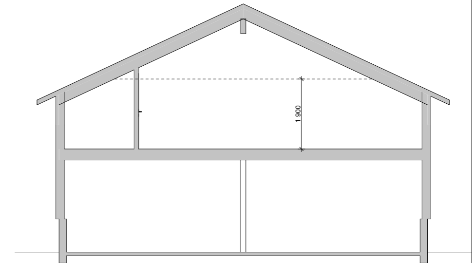
Snitt B 1:100
