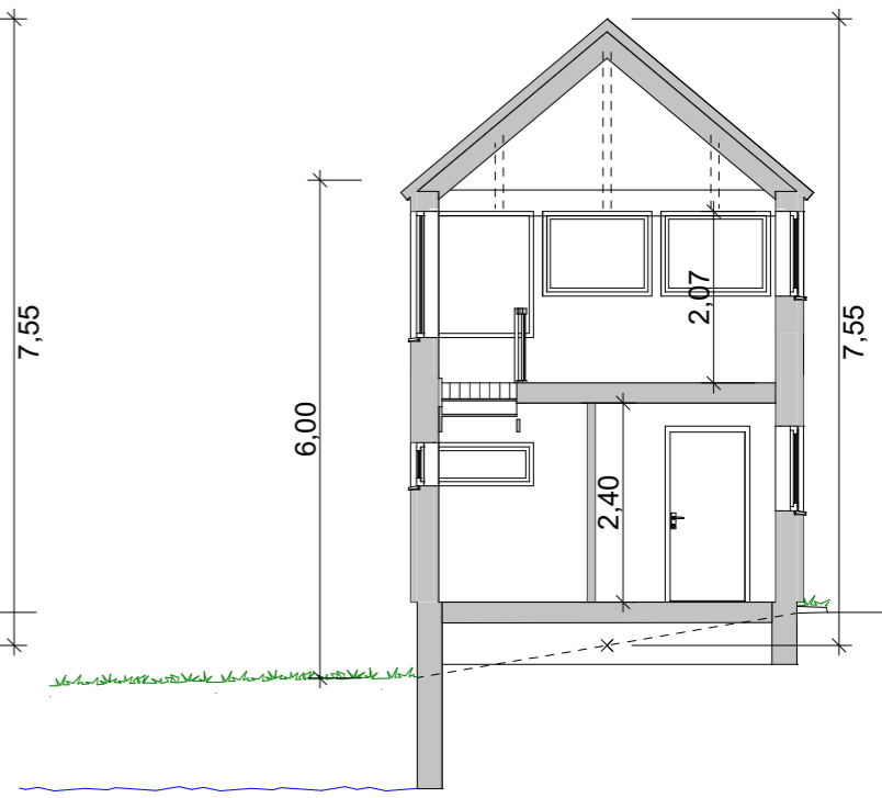
Snitt A-A
