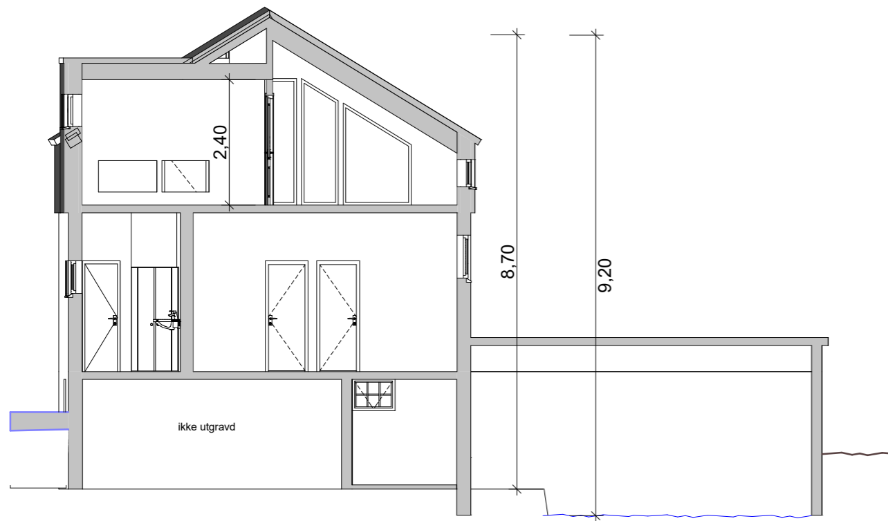
Snitt C-C
