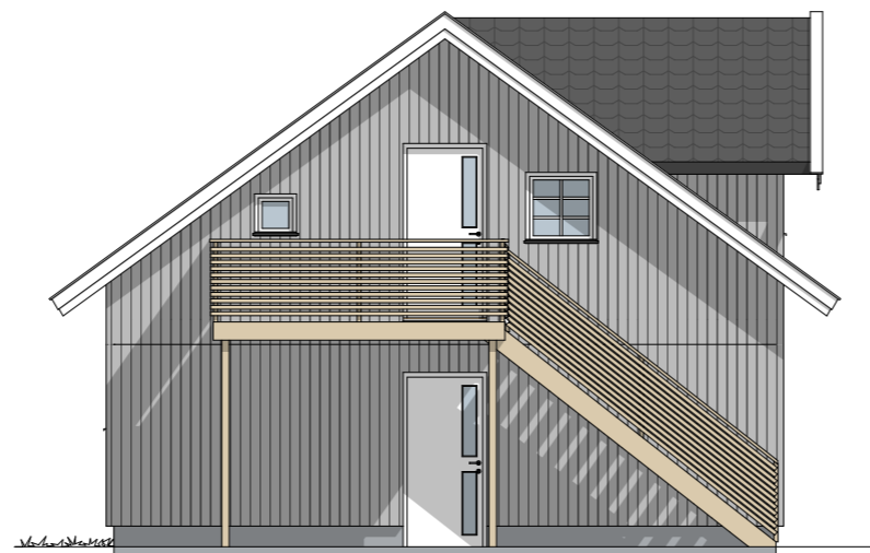
Fasade Nord 1:100
