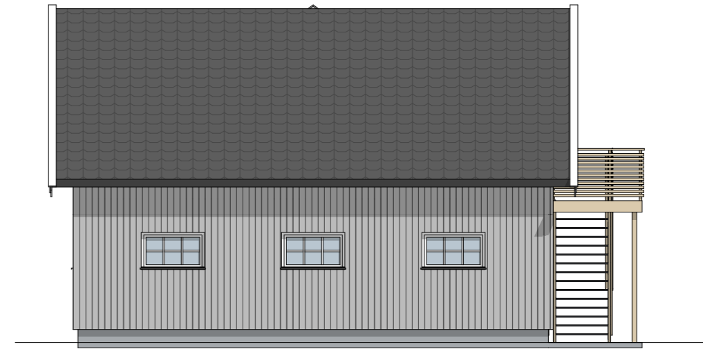
Fasade Øst 1:100
