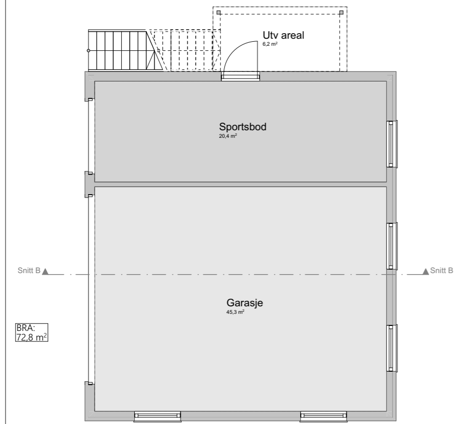
Plan 1. etasje 1:100
