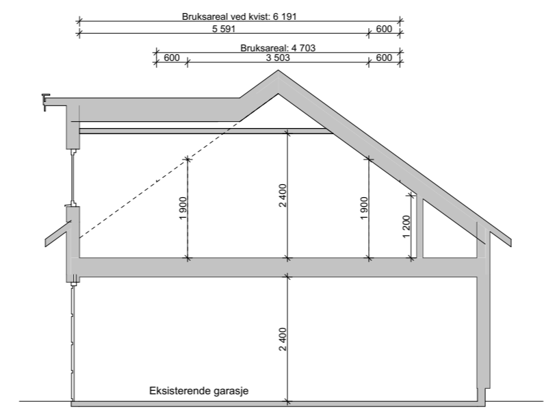
Snitt B 1:100
