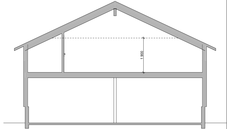
Snitt B 1:100
