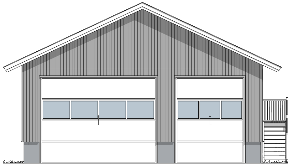
Fasade Nord 1:100
