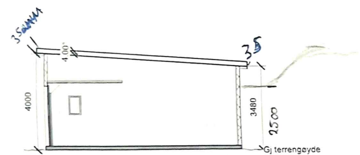
2 Snitt 1 : 100
