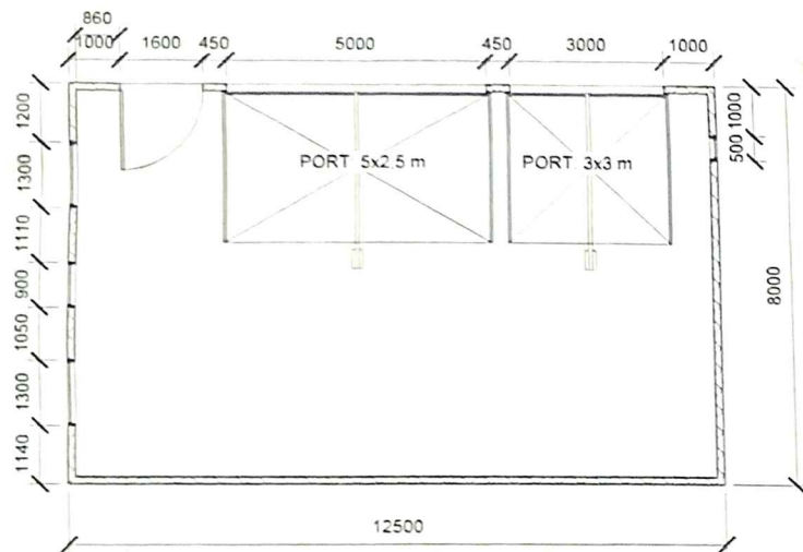
1 1. Plan 1 : 100
