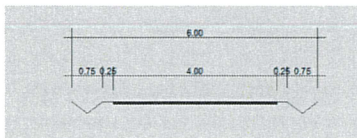
Figur 6 Normalprofil A1
