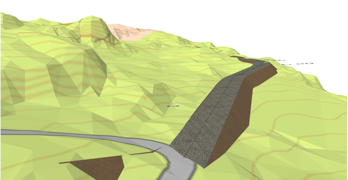
Figur 3. 3D-illustrasjon – perspektiv 2.
