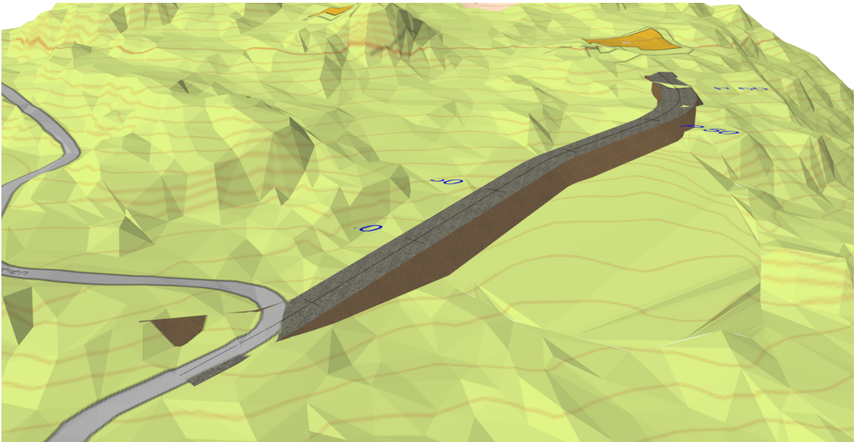
Figur 2. 3D-illustrasjon – perspektiv 1.
