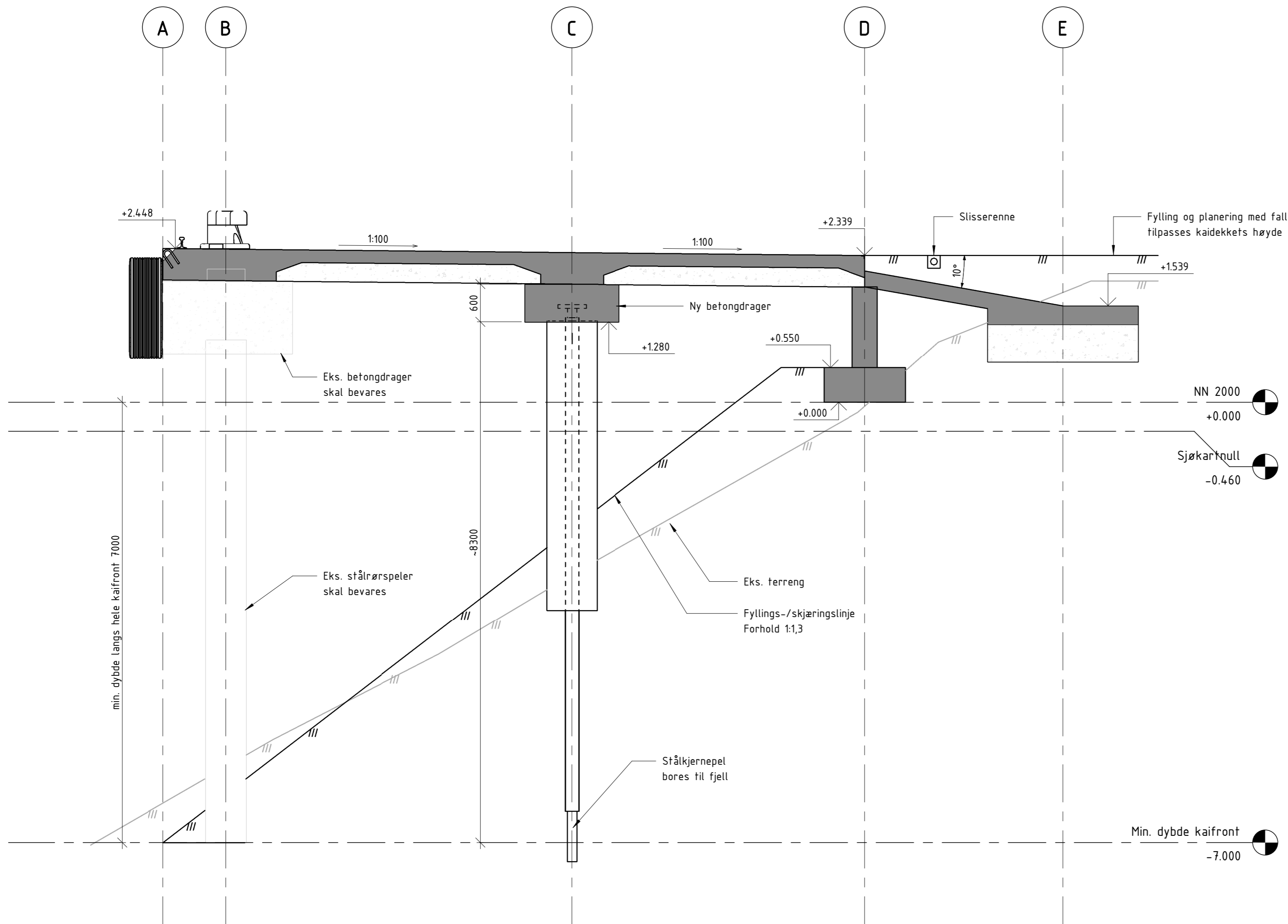
Snitt 14 - prinsipp 1 : 50
