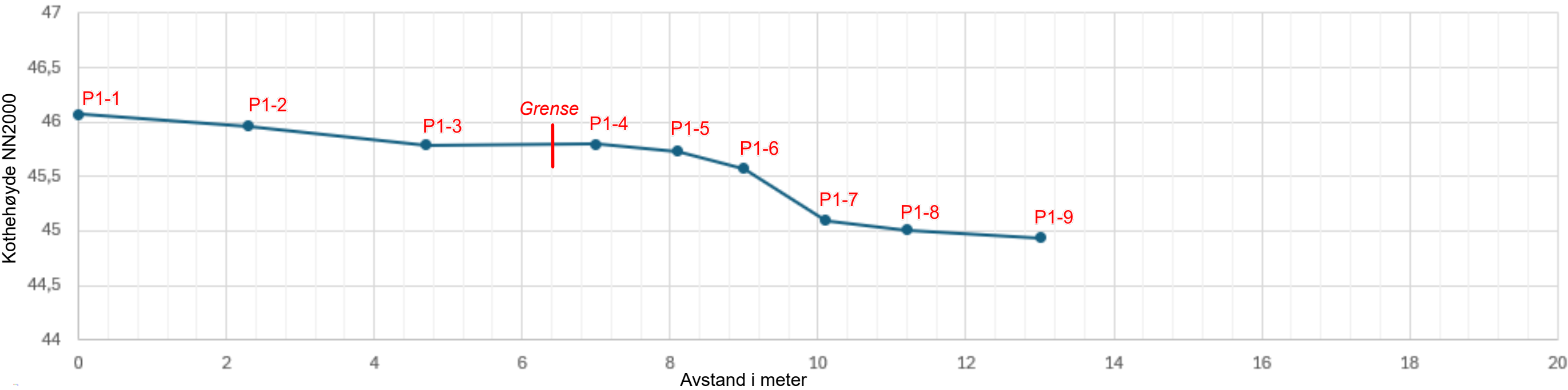
Terrengsnitt 1 1:1
