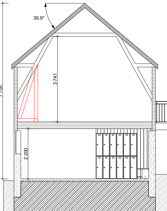
Snitt B 1:100
