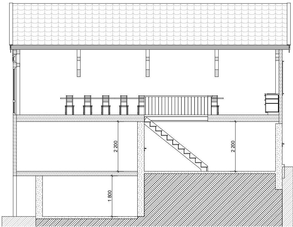
Snitt A 1:100
