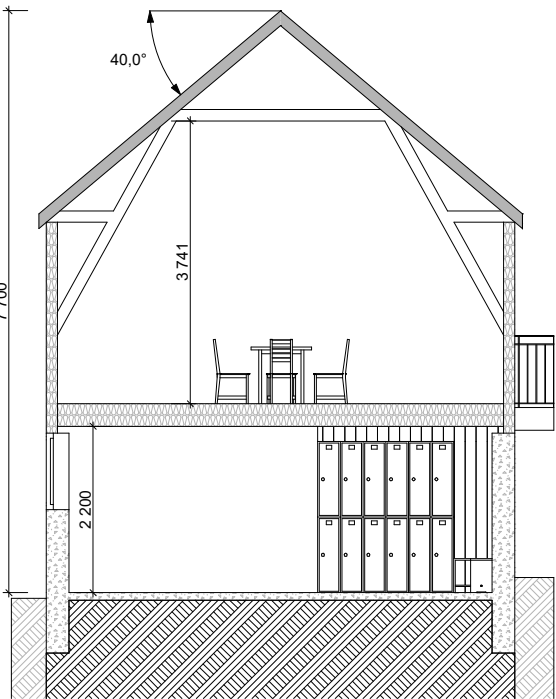
Snitt B 1:100
