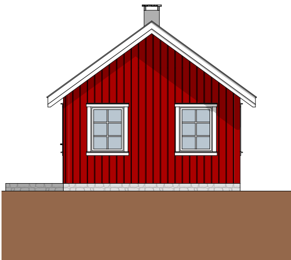
Fasade vest 1:100
