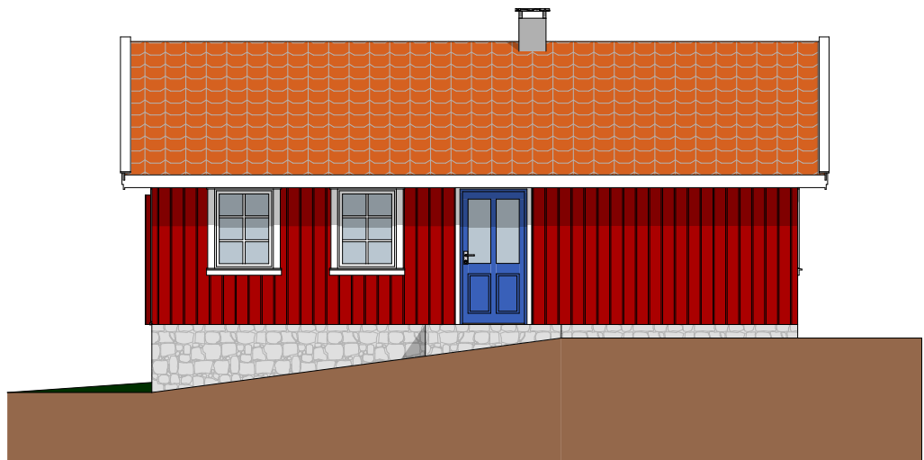
Fasade nord 1:100
