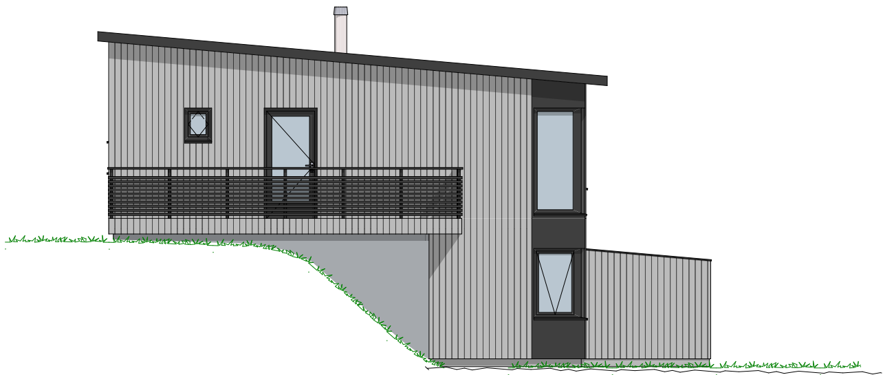
Fasade mot Sør-sør-vest
