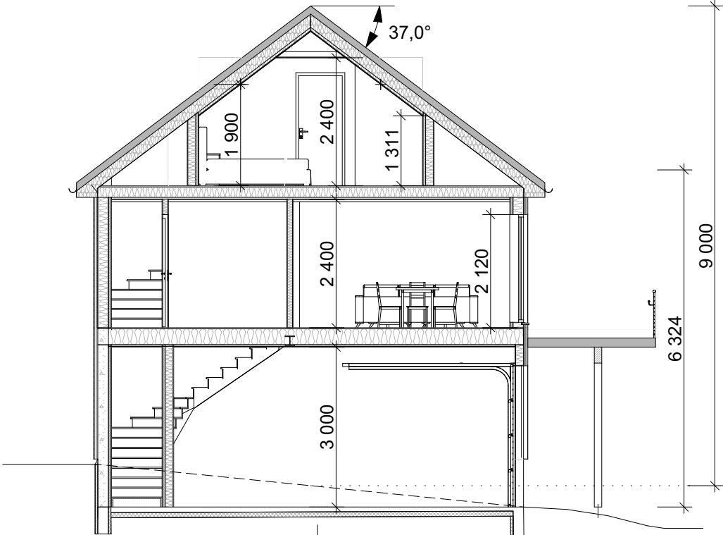
Snitt A-A
