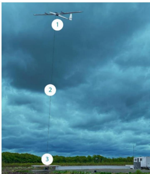
Figur 3: AMW system. 1: Kite, 2: line, 3: bakkestasjon. Kilde: Kitemill AS
