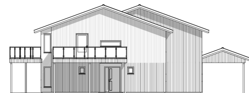
Fasade Vest
