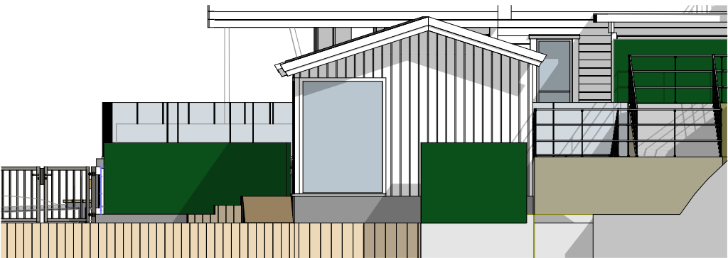
Fasade Fellesbygg 1:100
