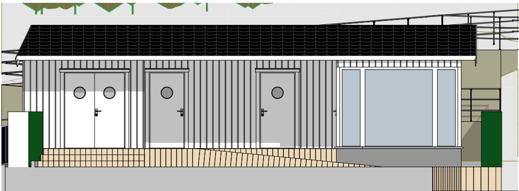
Fasade Fellesbygg 1:100
