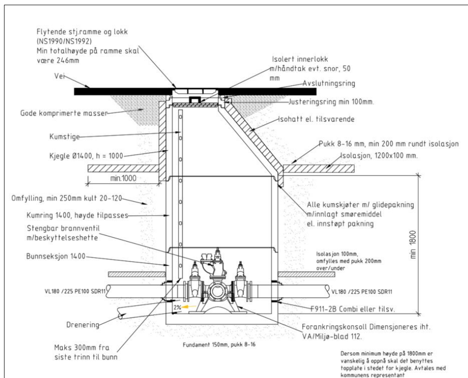
Figur 5-1. Standard oppbygging av kum med VL180-250 PE med stengbar brannventil.
