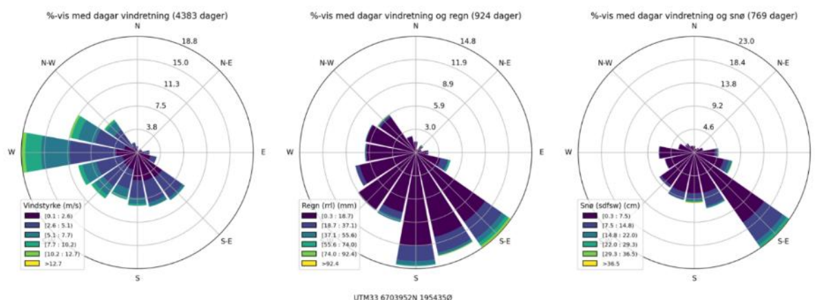
Figur 3-12: Vindroser frå Vardefjell (1121 moh.)
