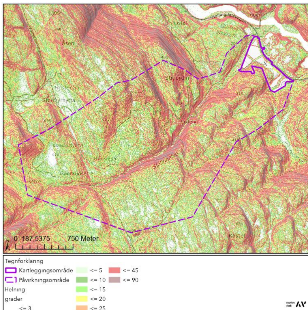
Figur 4-2: Terrenghellingskart tilpassa jord- og flaumskred.
