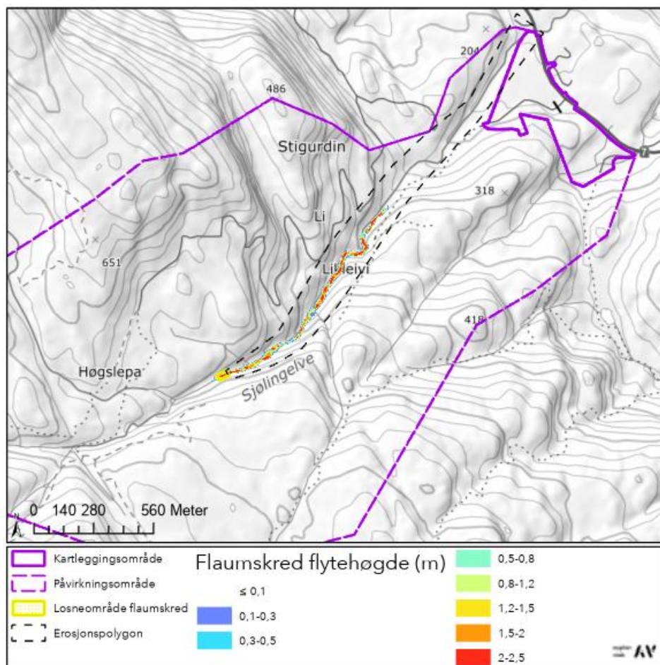
Figur 4-3: Modelleringsresultat for flaumskred vist med flytehogde. Viser at flaumskred stoppar før dei når kartleggingsområdet.
