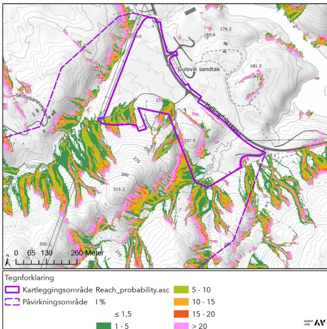
Figur 4-1: Simuleringsresultat RF3D vist med utløpssannsyn for området. Berre inkludert område som når inn i kartleggingsområdet, i utsnittet.
