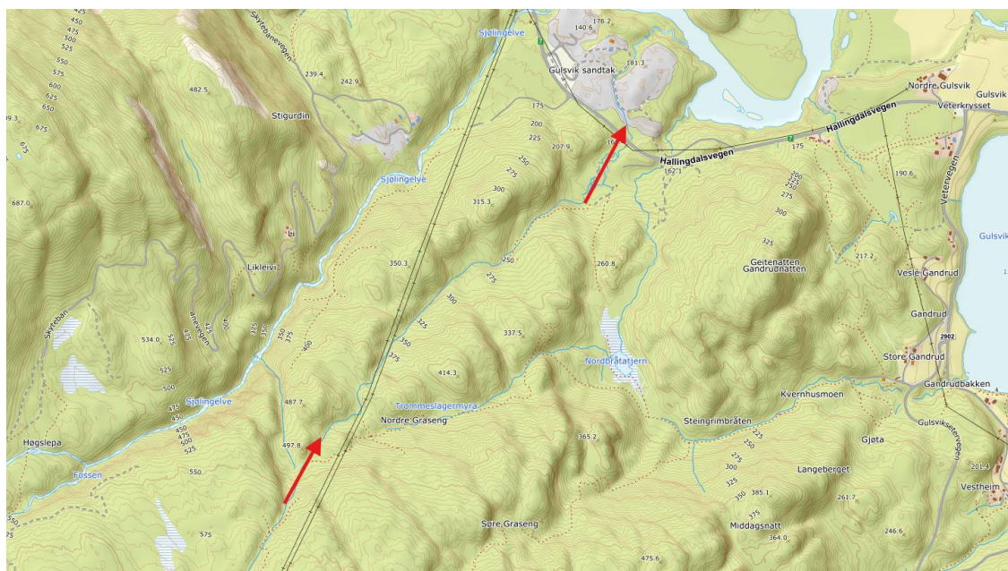
Figur 2-3. Fly- og lidarbilder indikerer at bekkeløpet fra Lauvhaugen har sitt løp mot nordøst og munner ut i Hallingdalselva etter å ha passert gjennom Gulsvik sandtak. Pilene illustrerer strømningsretningen som er lagt til grunn i vurderingene.
