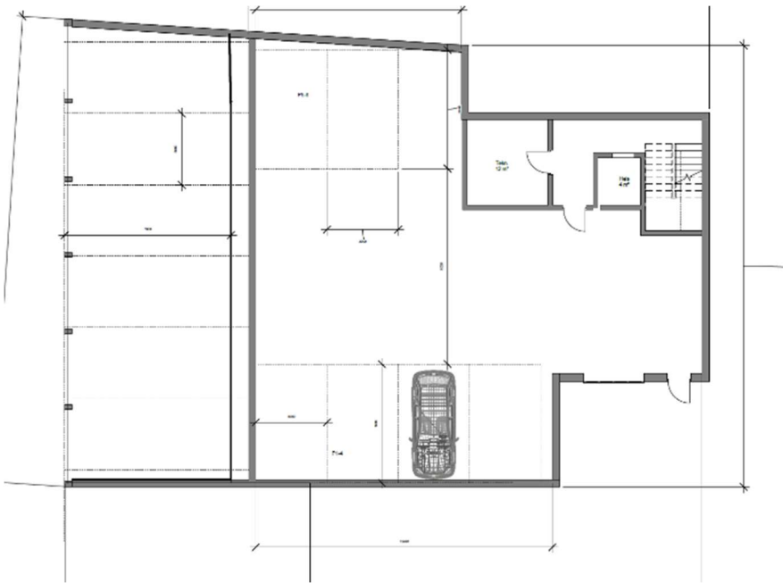
FIGUR 21: ILLUSTRASJON AV PARKERINGSLØSNING
