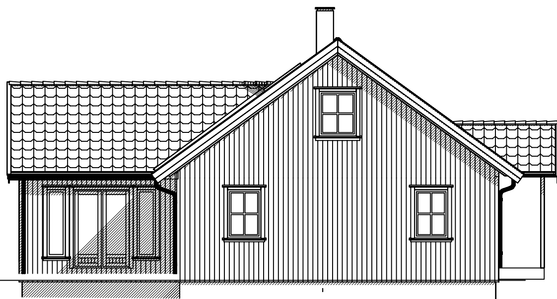
FASADE SØRØST
