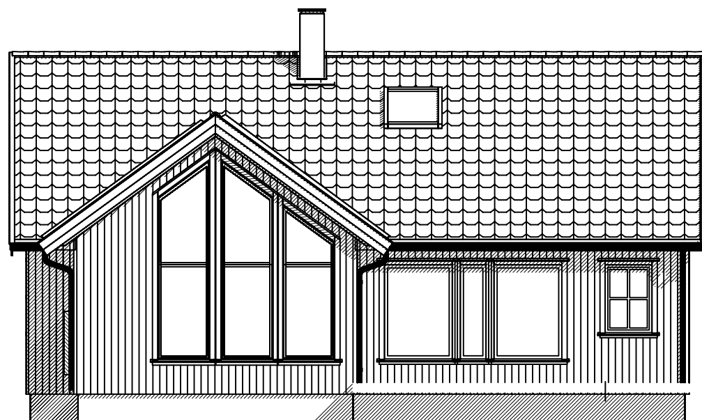
FASADE SØRVEST
