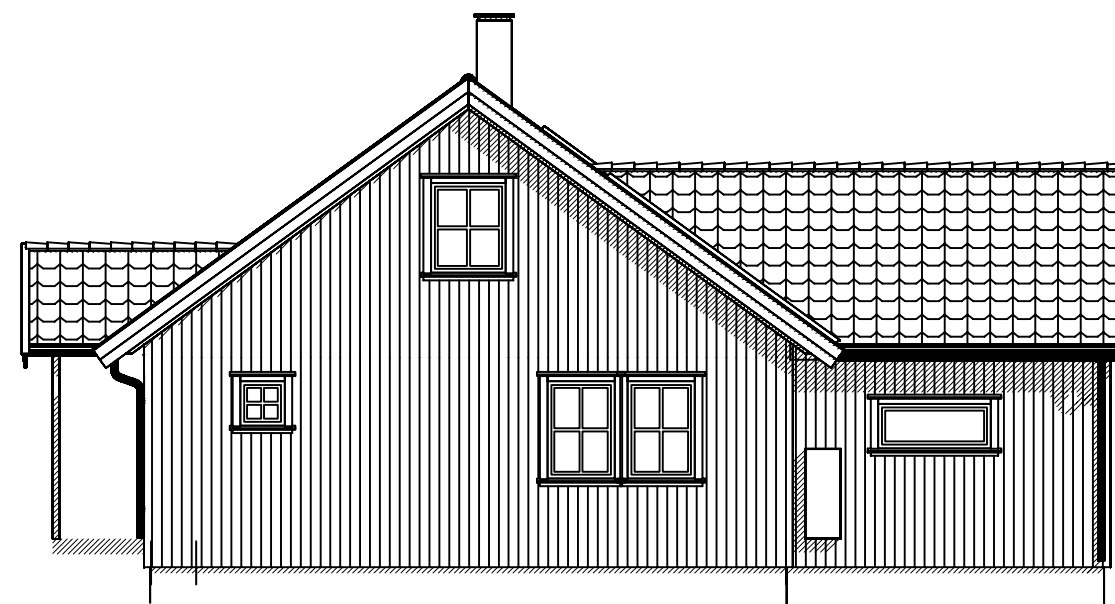
FASADE NORDVEST
