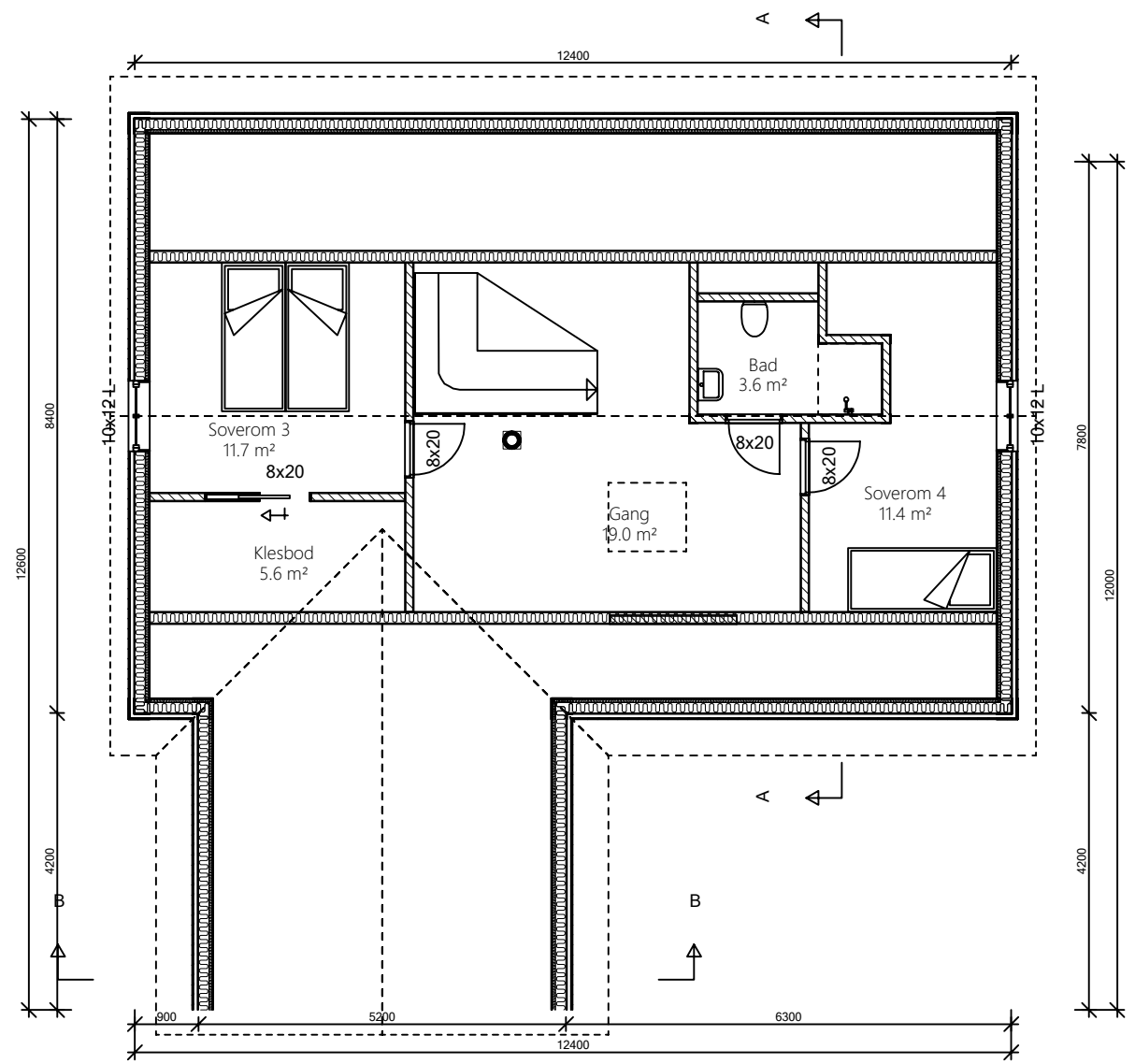
Plan loft
