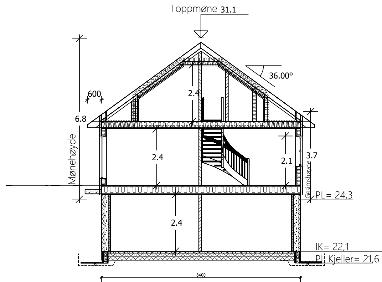
SNITT A-A
