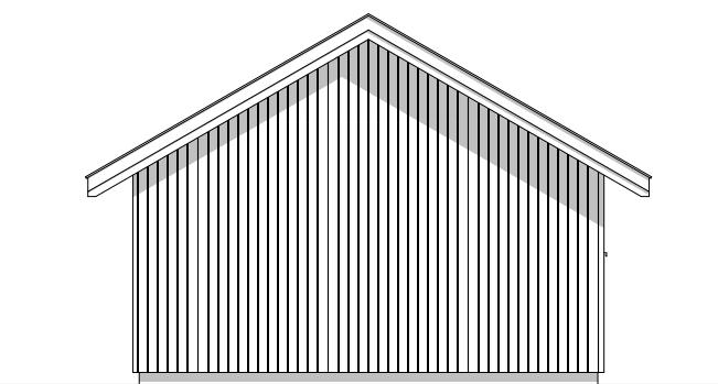
Fasade nordvest
