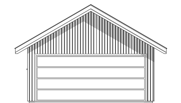
Fasade sydøst
