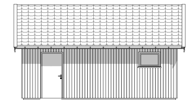
Fasade sydvest
