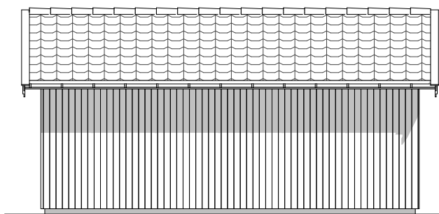
Fasade nordøst
