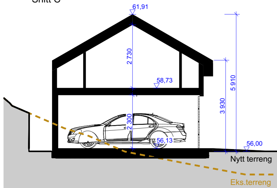
Snitt C
