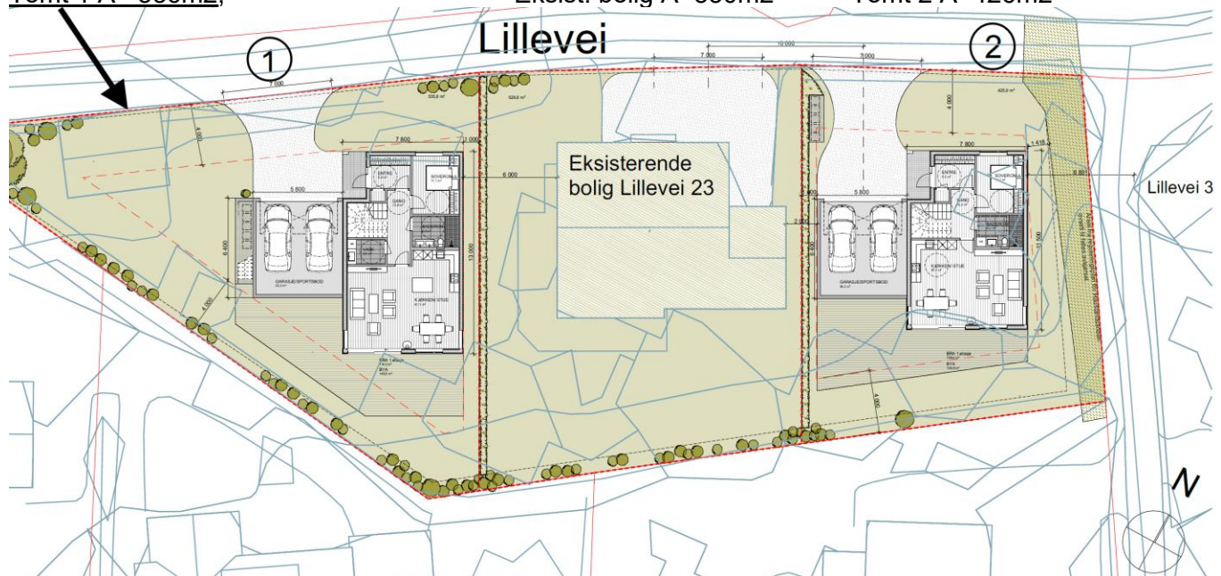
Situasjonsplan
