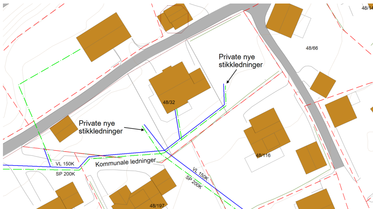
Skisse for eksisterende og nytt ledningsanlegg.
