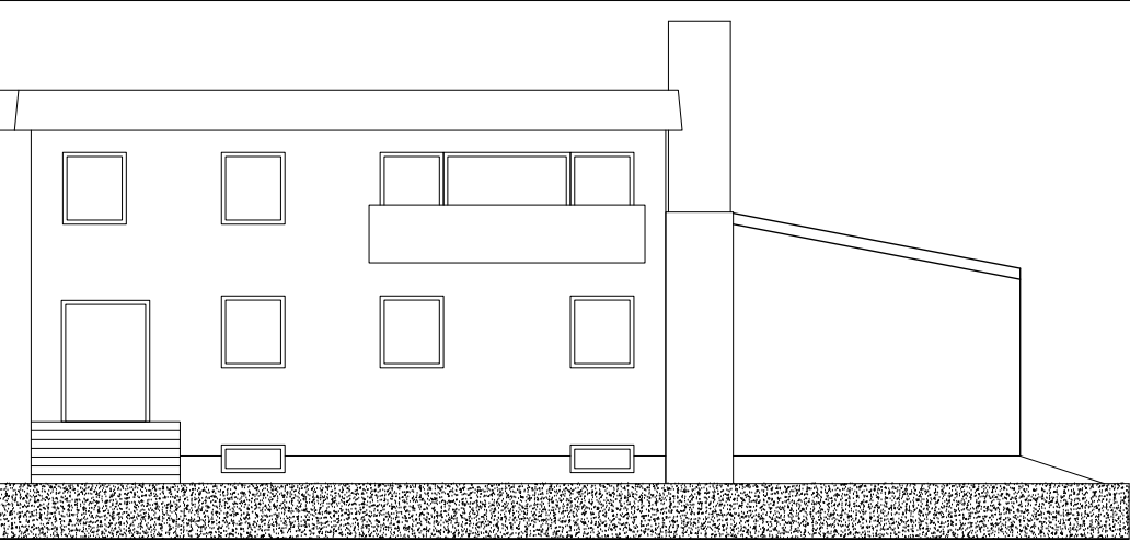
Nord-Vest
