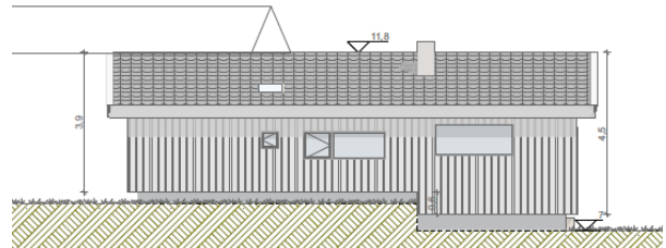
Fasade Vest
