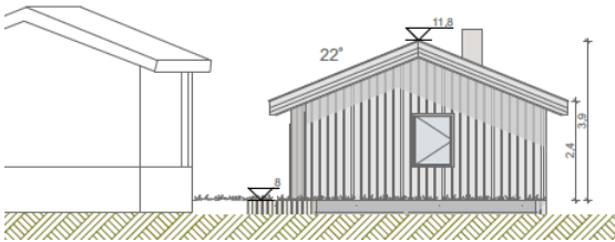
Fasade Øst
