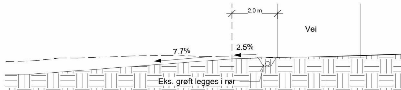
Snitt avkjørsel 1 : 100
