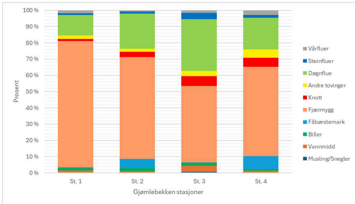
Figur 3. Prosentvis fordeling av bunndyrgrupper på de ulike stasjonene i Gjømlbekken.
