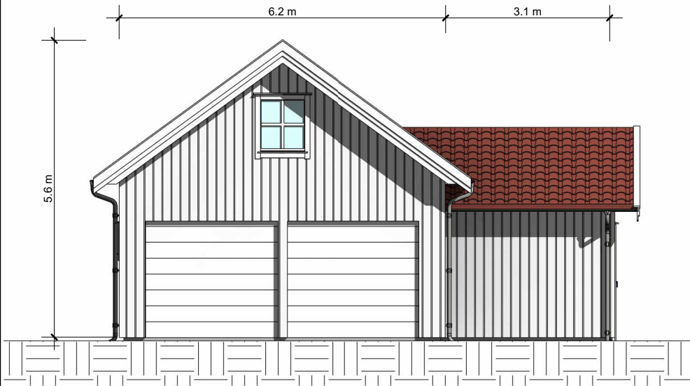
Fasade Sør 1 : 100
