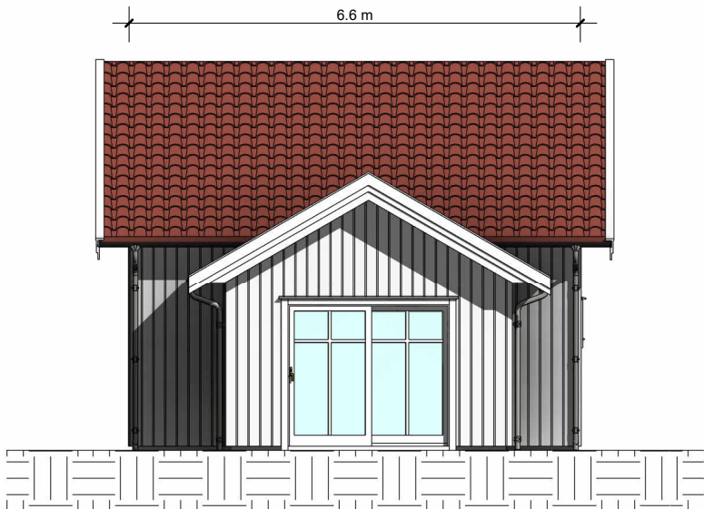
Fasade Øst 1 : 100
