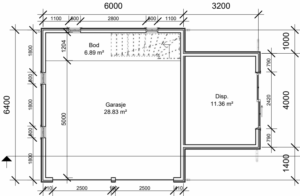
Plan 1. Etg 1 : 100
