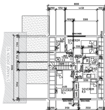
PLAN 2. ETASJE
