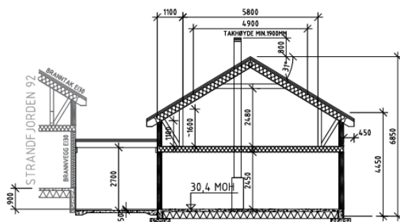
SNITT FUNDAMENTERING OG DRENERING VURDERES UT FRA STEDLIGE FORHOLD.
