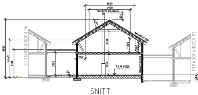
Snittegning
