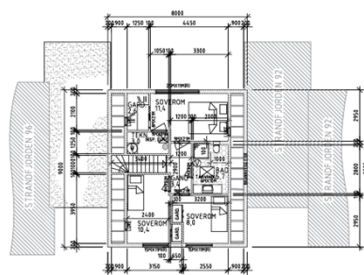
PLAN 2. ETASJE
