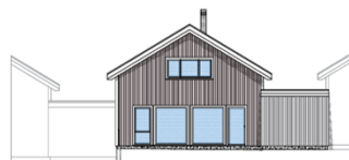
FASADE MOT NORDVEST
