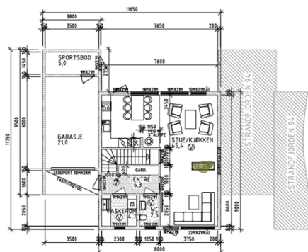
PLAN 1. ETASJE
