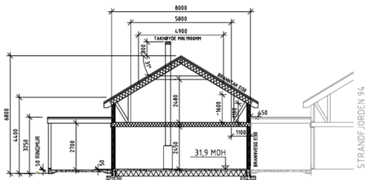
SNITT
