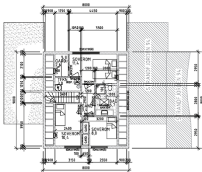
PLAN 2. ETASJE
