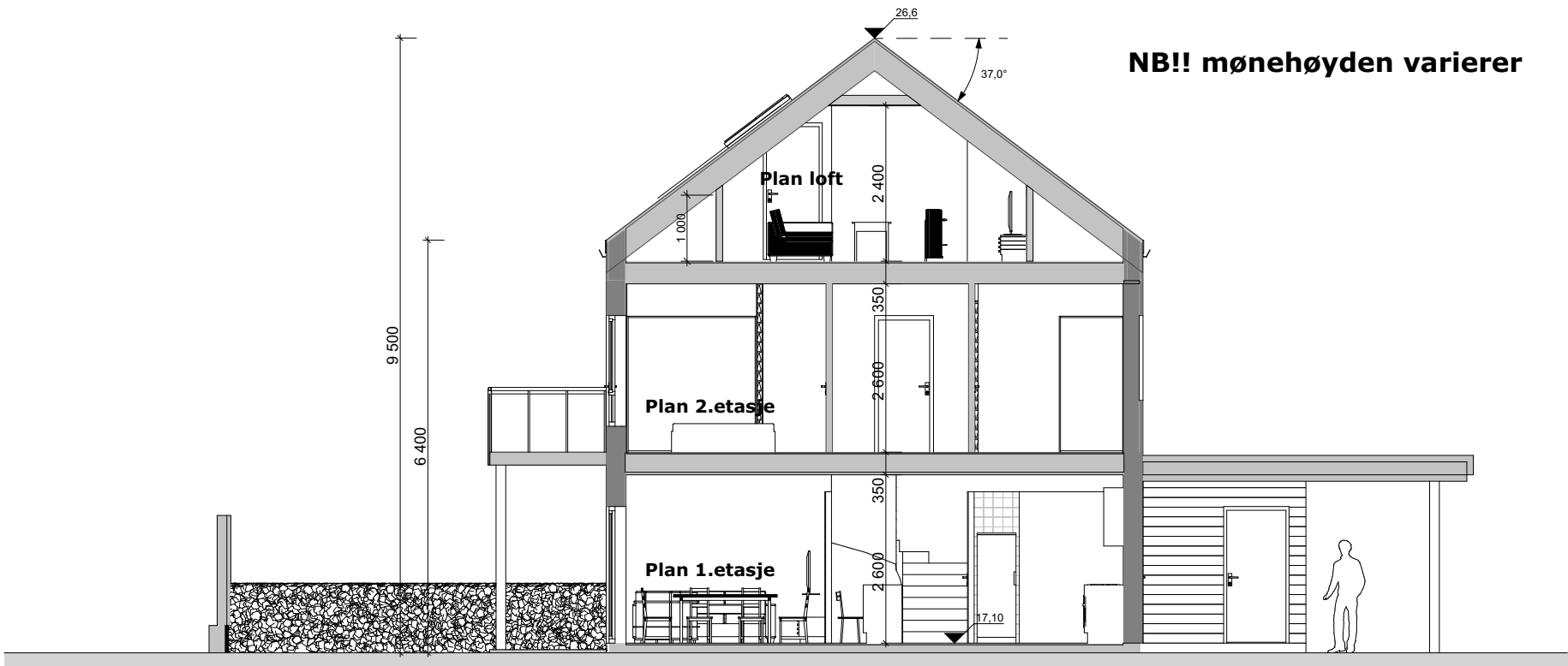
Snitt tomannsbolig - 1:100
