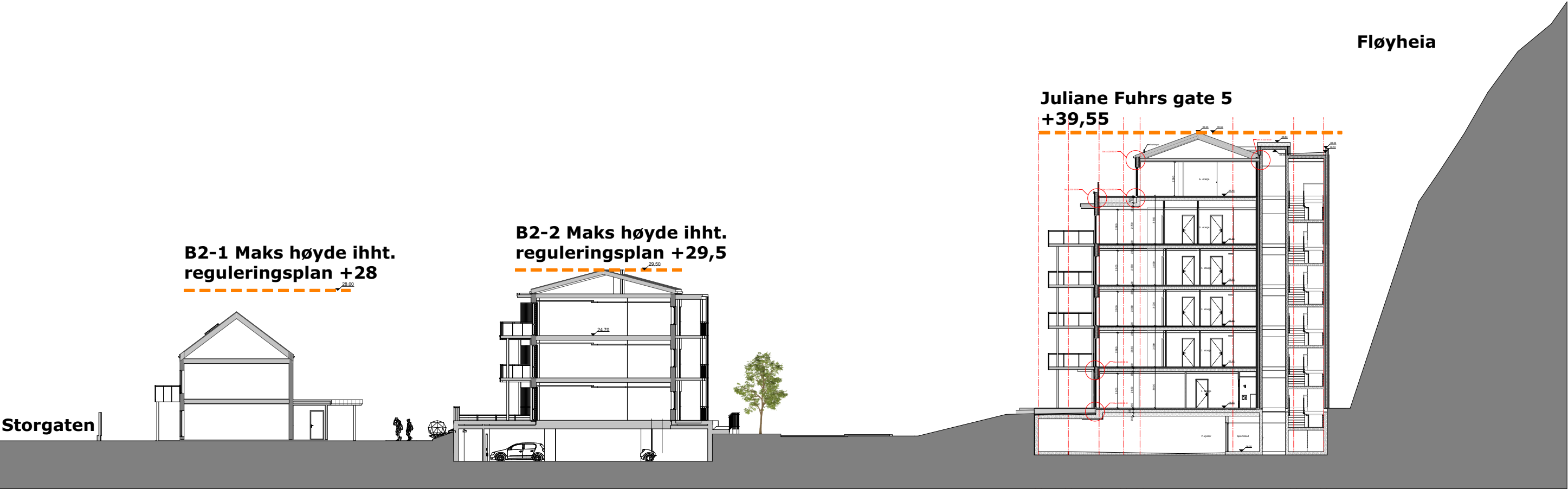
Snitt CC - 1:300
