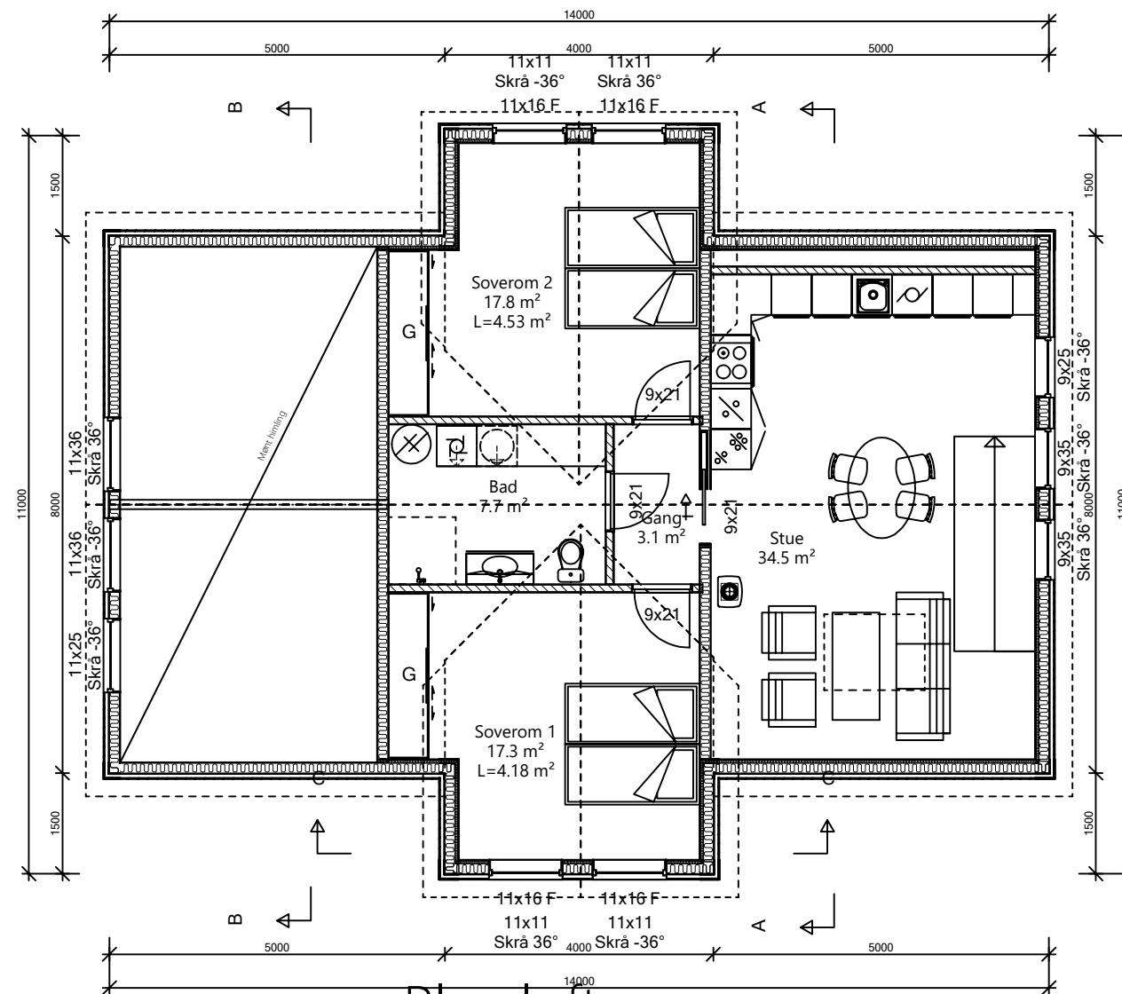
Plan loft
