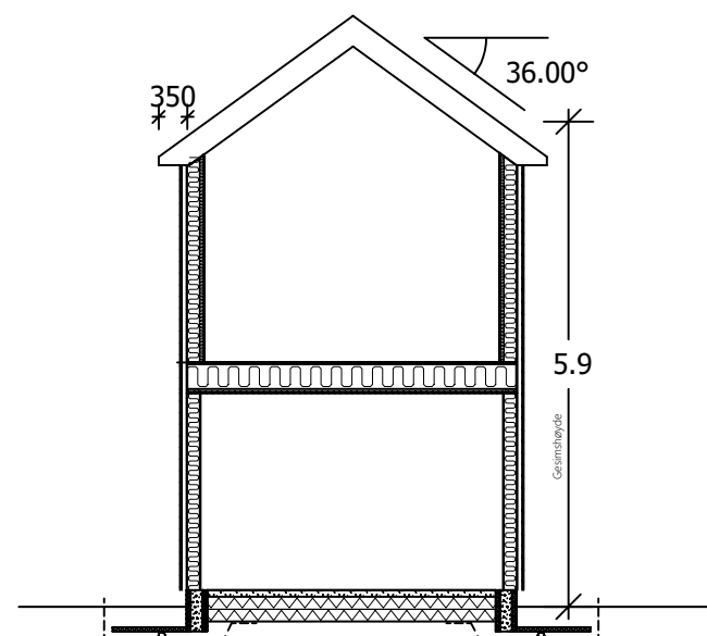
SNITT C - C
