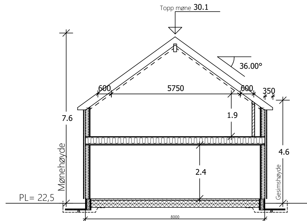
SNITT A - A
