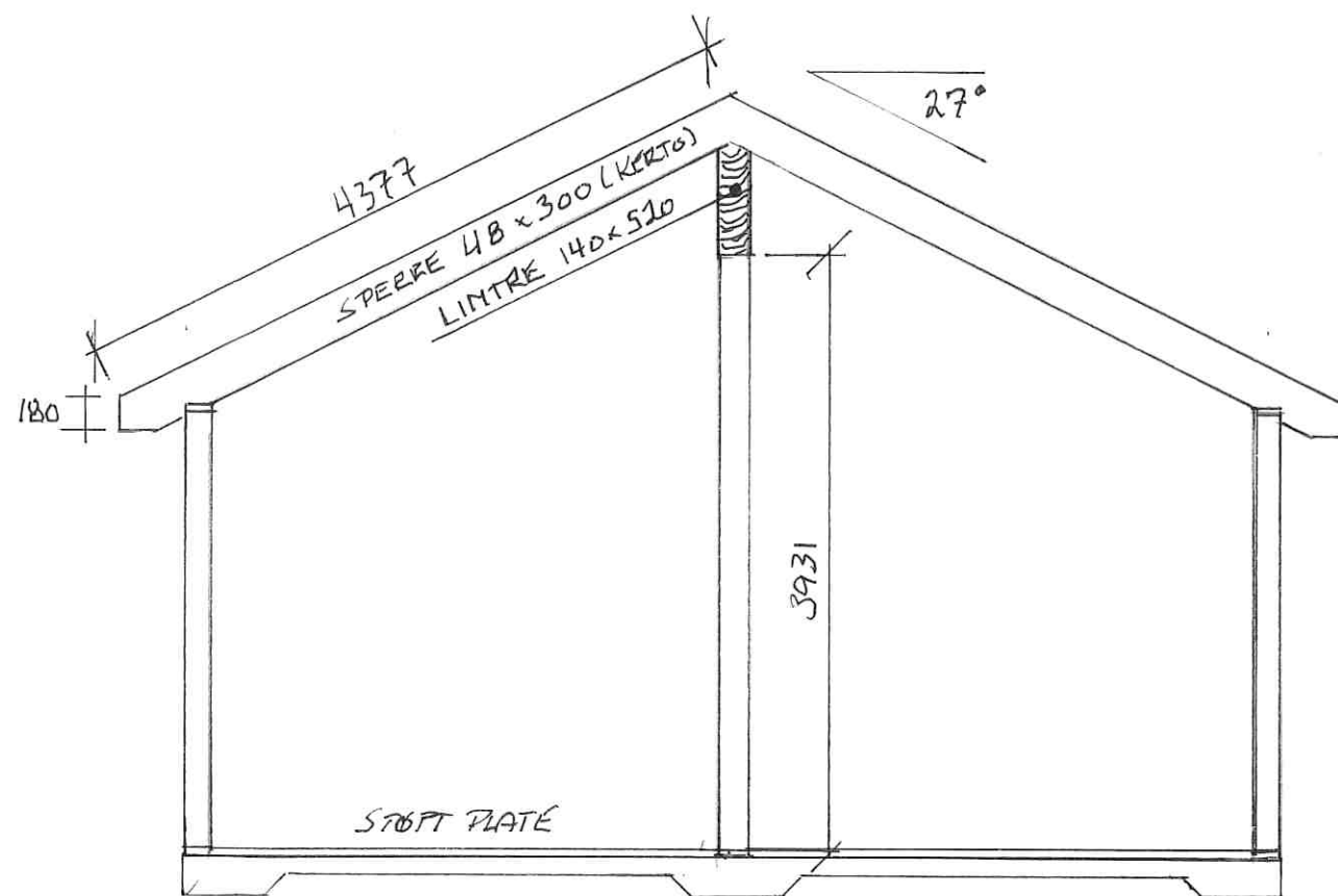
SNITT B-B
