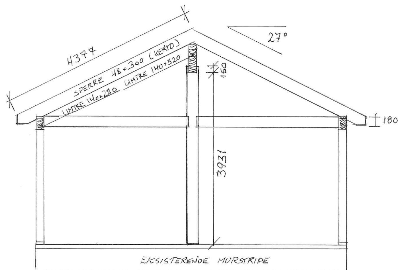
SNITT A-A
