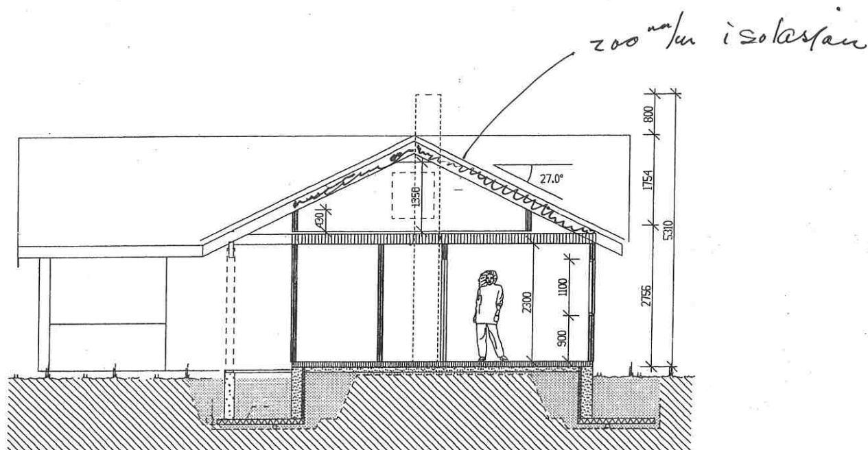
SNITT A/A
