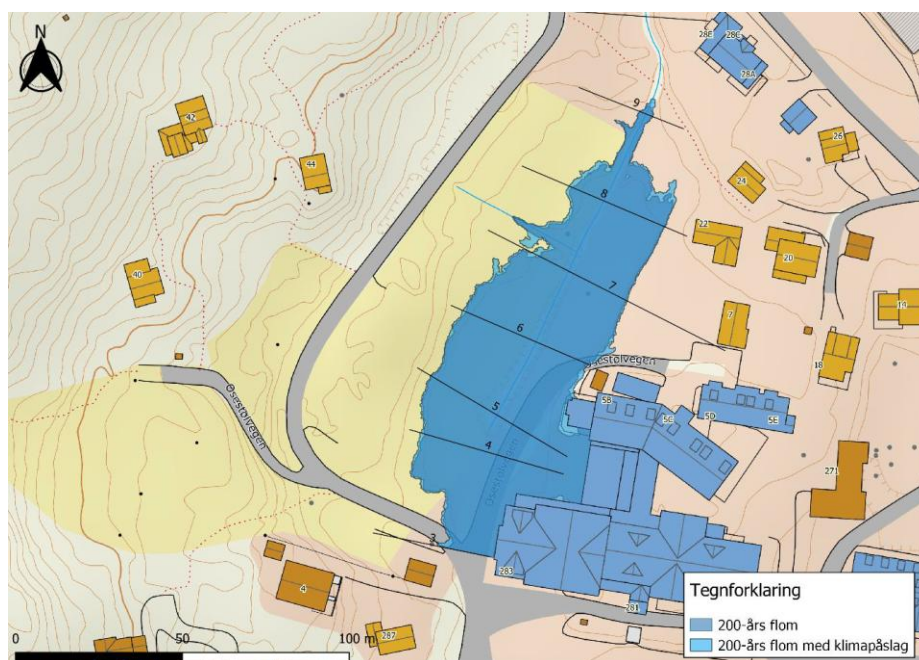
Figur 5: Flomsonekart som viser utbredelsen ved 200-års flom med og uten klimapåslag
