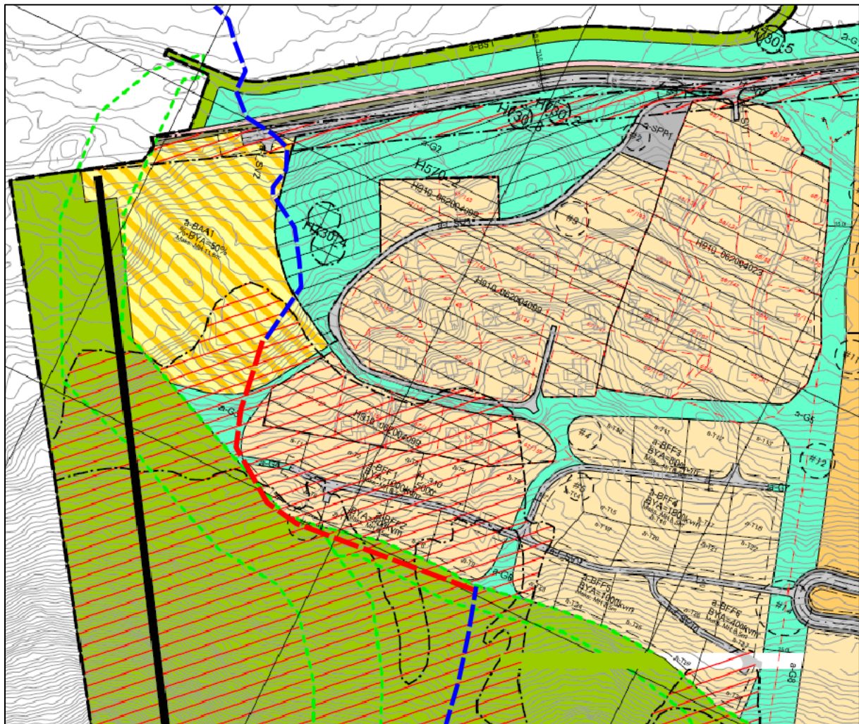
Figur 4: Eksisterende trase til Bekk 4 (blå) og foreslått ny trase (rød).
