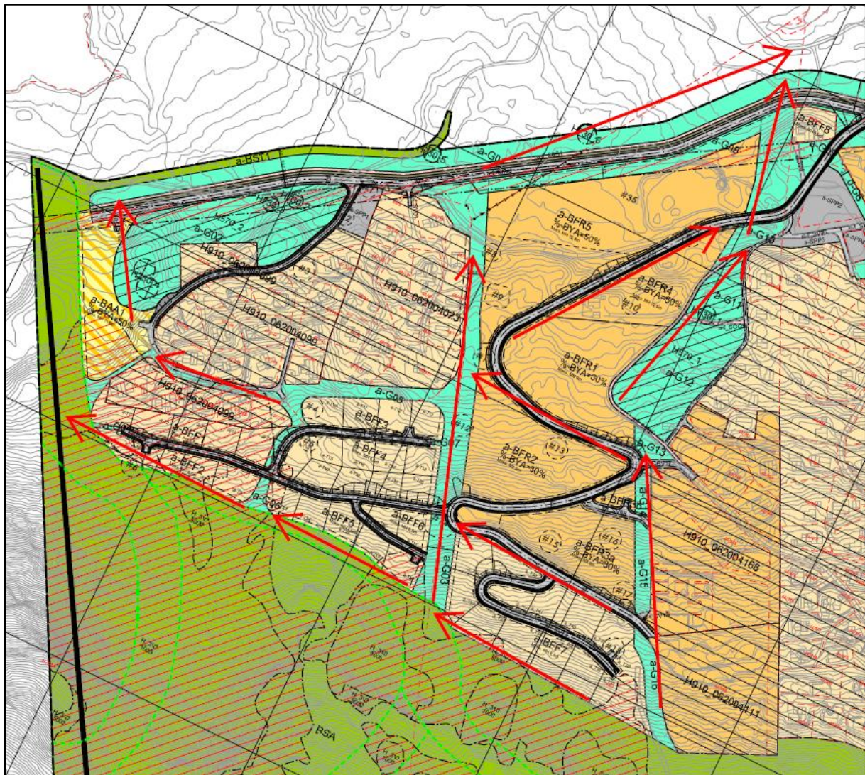
Figur 6. Området vest. Det etablere avskjærende grøfter oppstrøms utbyggingsområdene, og det lages sikre overvanns- og flomløp til Ustedalsfjorden. I tillegg vil en få avskjæring av området med alle planlagte veger, slik at en får en trygg bortledning av overflatevann og ekstra sikkerhet ved flomsituasjoner.
