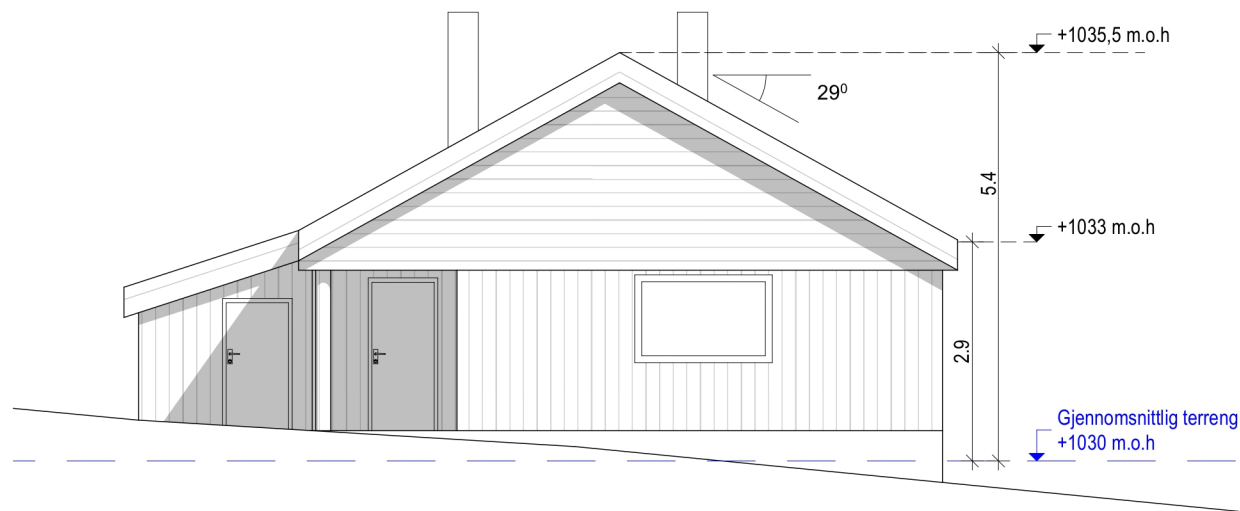
Sørvest (1:100)
