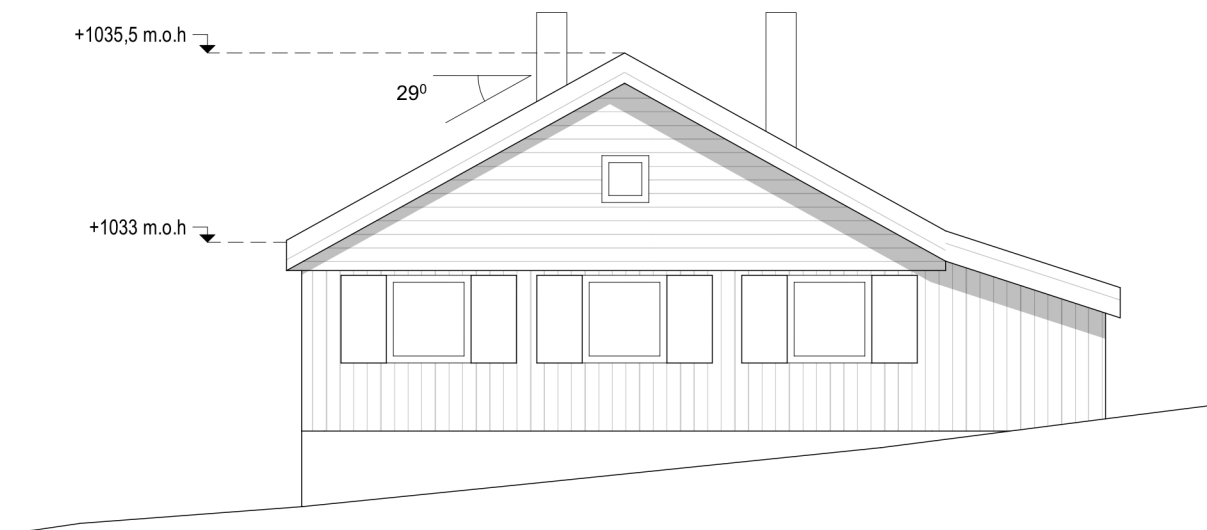
Nordøst (1:100)
